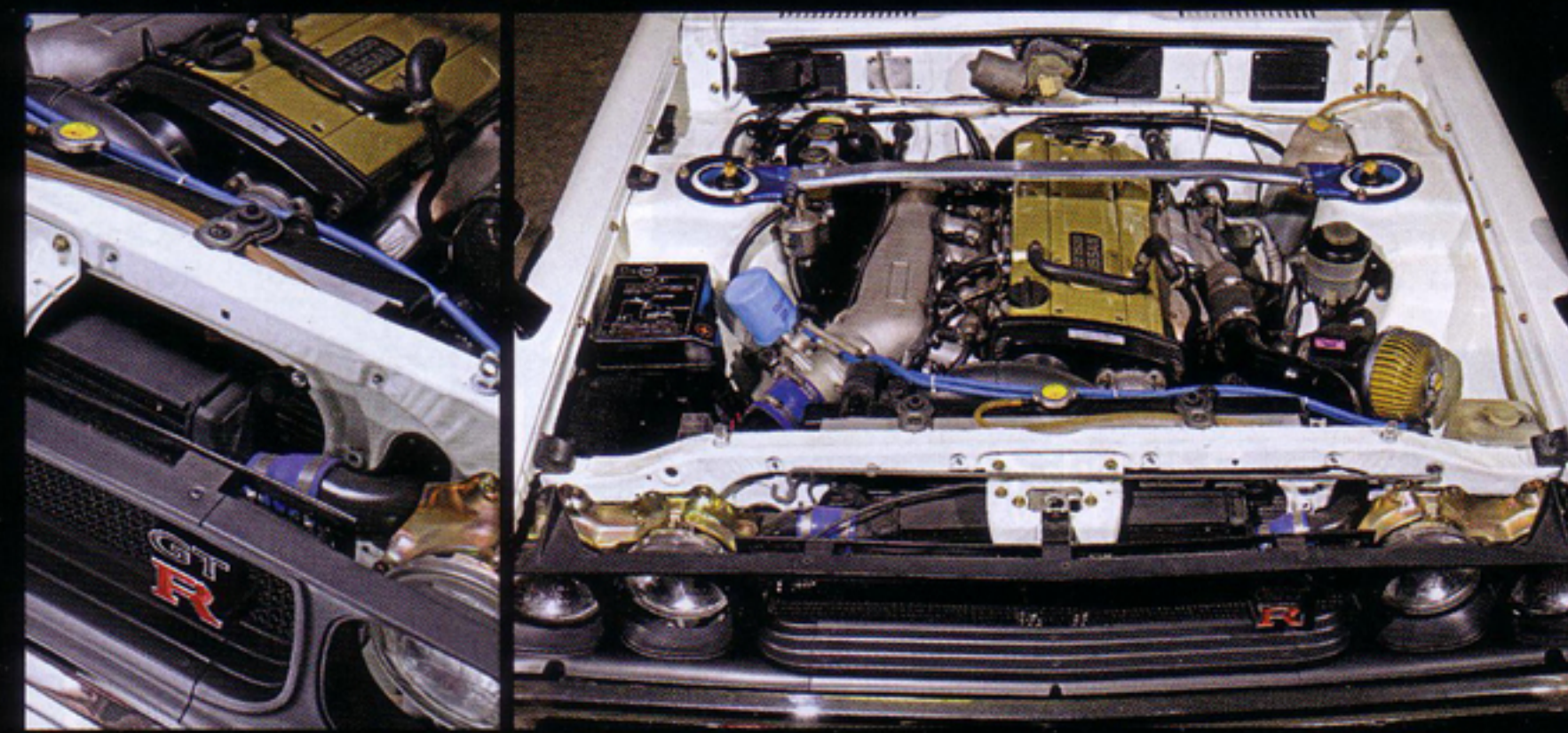
エンジンはR33スカイライン用のRB25DETをライトチューン。レイアウト性を向上させるために、トラストのサージタンクなどを使用している。グリル内のスペースにブラックアウトしたインタークーラーを装着。外観的にはあくまでも当時ふうの仕上げを目指す。
